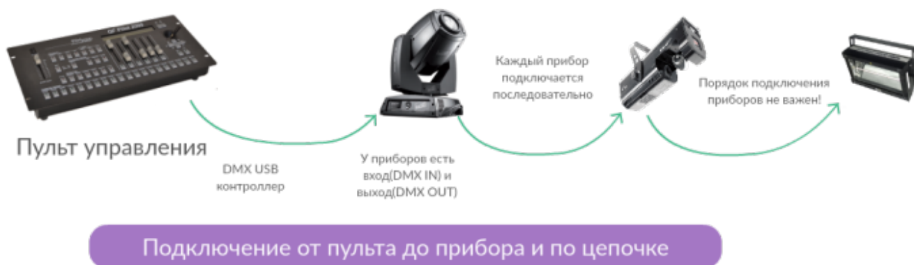
Схема построения DMX 512 сети используя пульт управления
